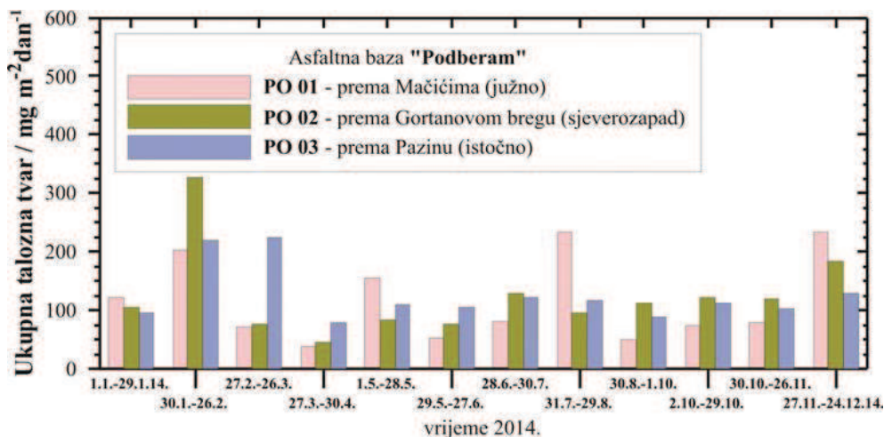
Slika 9. Kretanje mjesečnih količina ukupnih taložnih tvari za razdoblje u 2014. godini
