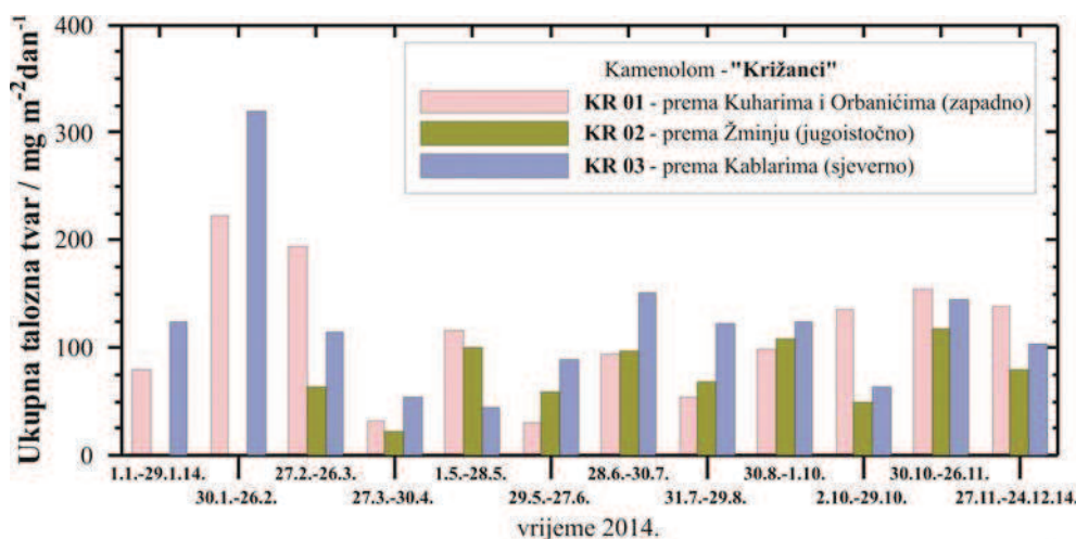
Slika 8. Kretanje mjesečnih količina ukupnih taložnih tvari za razdoblje u 2014. godini
