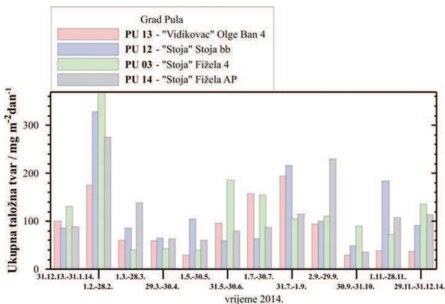
Slika 5b. Kretanje mjesečnih količina ukupnih taložnih tvari za razdoblje u 2014. godini
