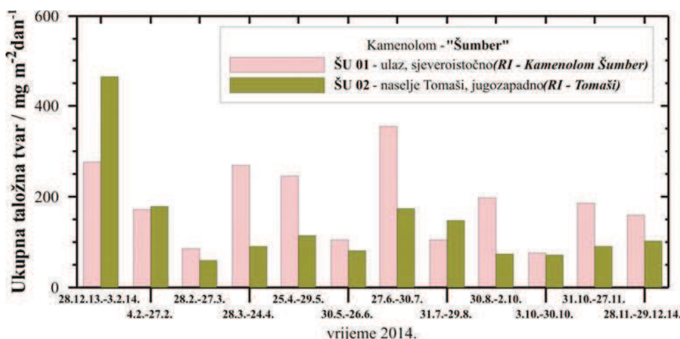
Slika 12. Kretanje mjesečnih količina ukupnih taložnih tvari za razdoblje u 2014. godini
