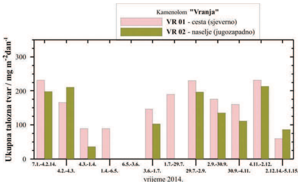
Slika 13. Kretanje mjesečnih količina ukupnih taložnih tvari za razdoblje u 2014. godini
