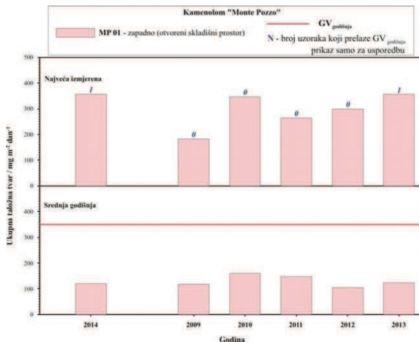
Slika 28. Usporedba rezultata mjerenja ukupne taložne tvari sa kriterijima za vrednovanje kvalitete zraka na mjernejoj postaji MP 01
