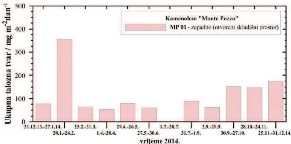
Slika 14. Kretanje mjesečnih količina ukupnih taložnih tvari za razdoblje u 2014. godini
