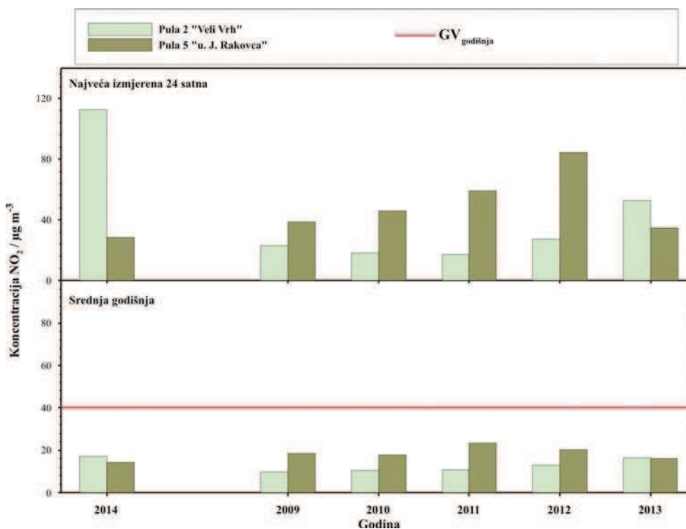
Slika 18. Usporedba rezultata mjerenja dušikova dioksida sa kriterijima za vrednovanje kvalitete zraka na području Grada Pule
